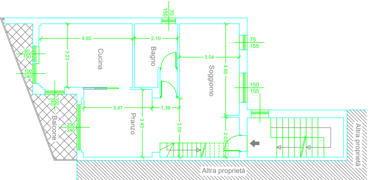
PIANTA PIANO PRIMO - PROGETTO
